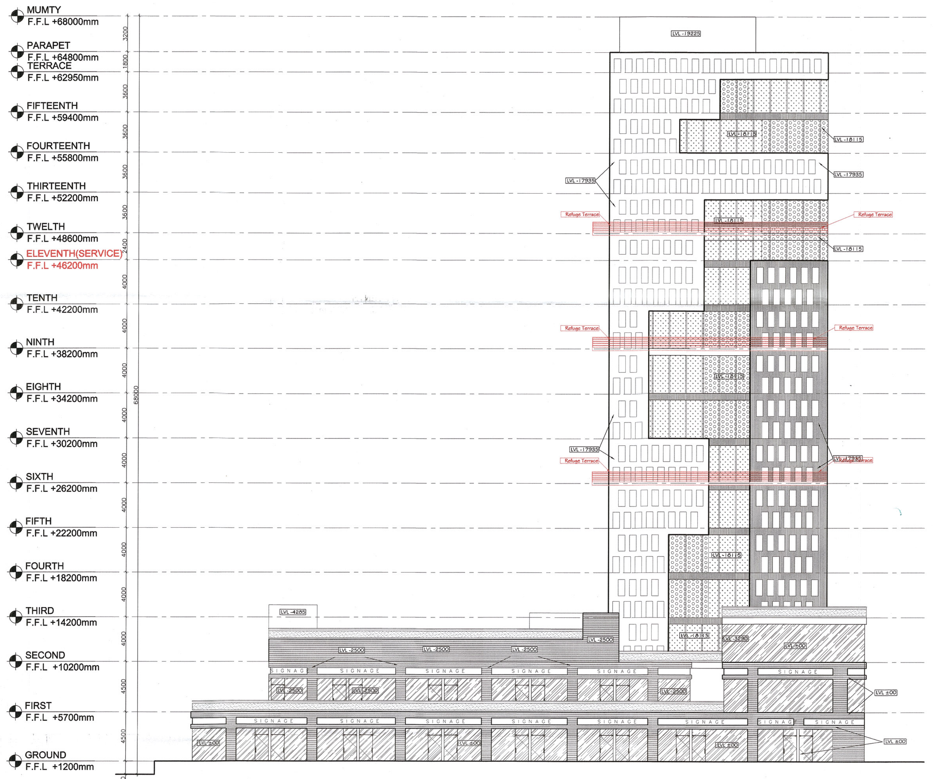
ELEVATION 4
