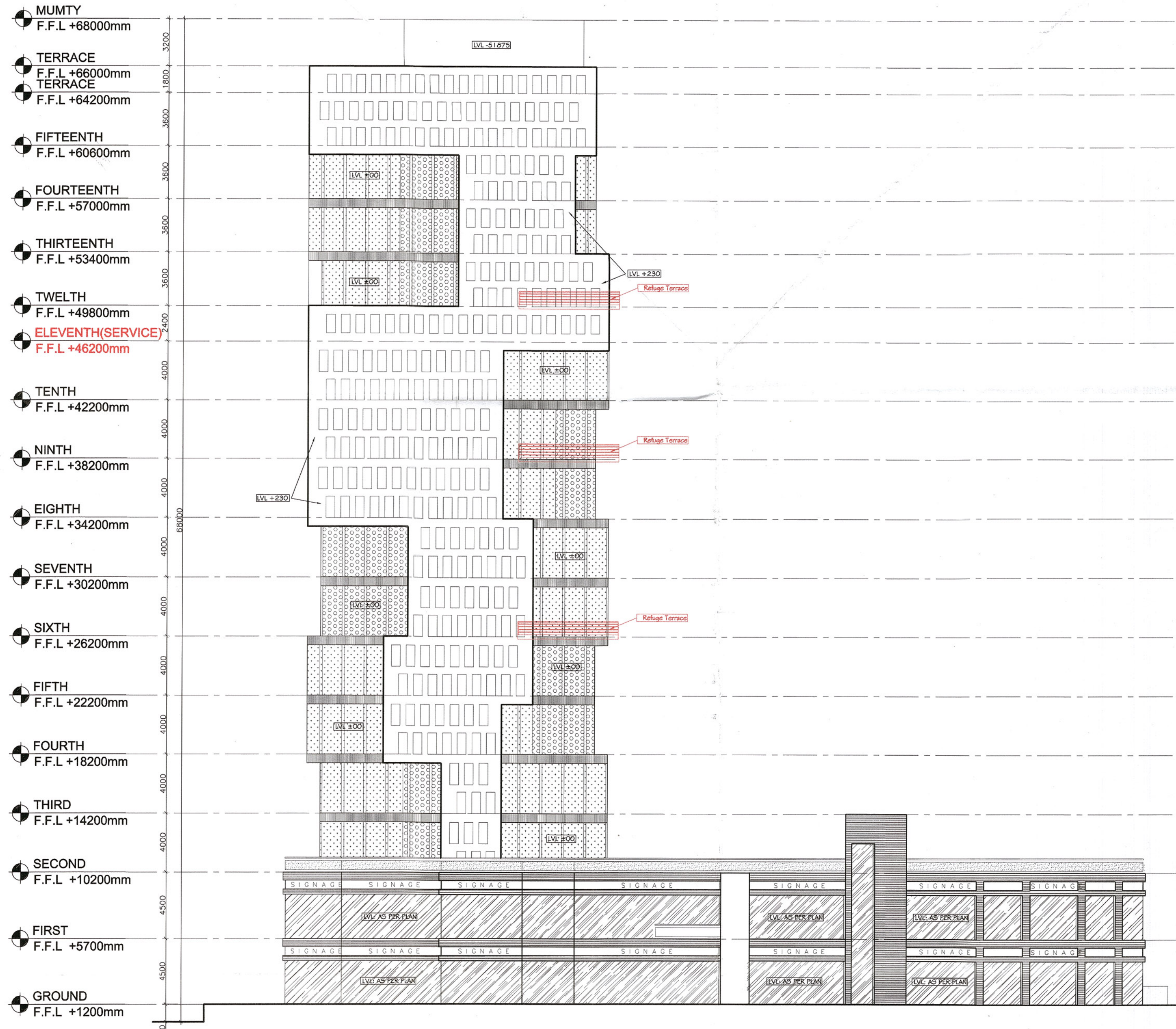
ELEVATION 2
